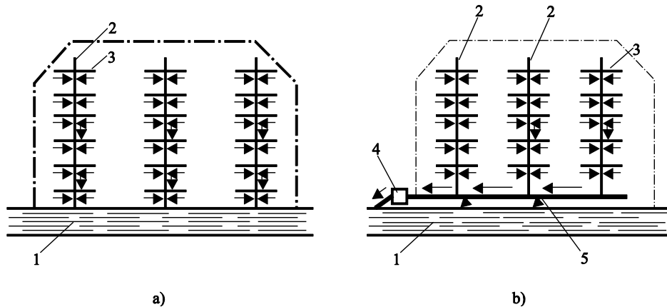
Figura 2. Schema perpendiculară: a – directă; b – indirectă
