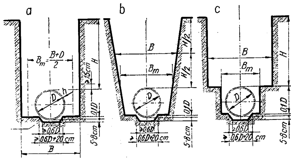
Fig. 1 Secțiuni de pozare uzuale tipizate
