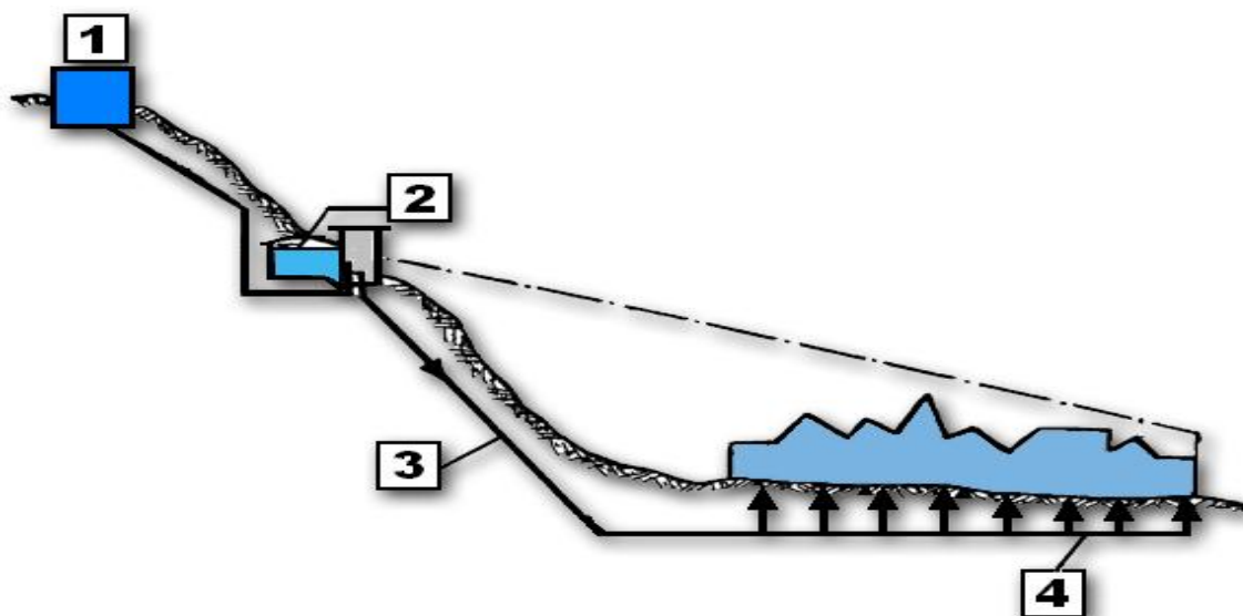
Figura 1.2. Schema alimentării cu apă, având ca sursă un izvor situat la cotă ridicată
