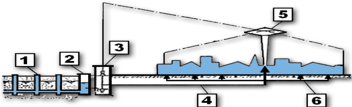
Figura 1.6. Schema alimentării cu apă, având ca sursă apa subterană captată prin puțuri sau drenuri și pomparea ei în castel de apă
